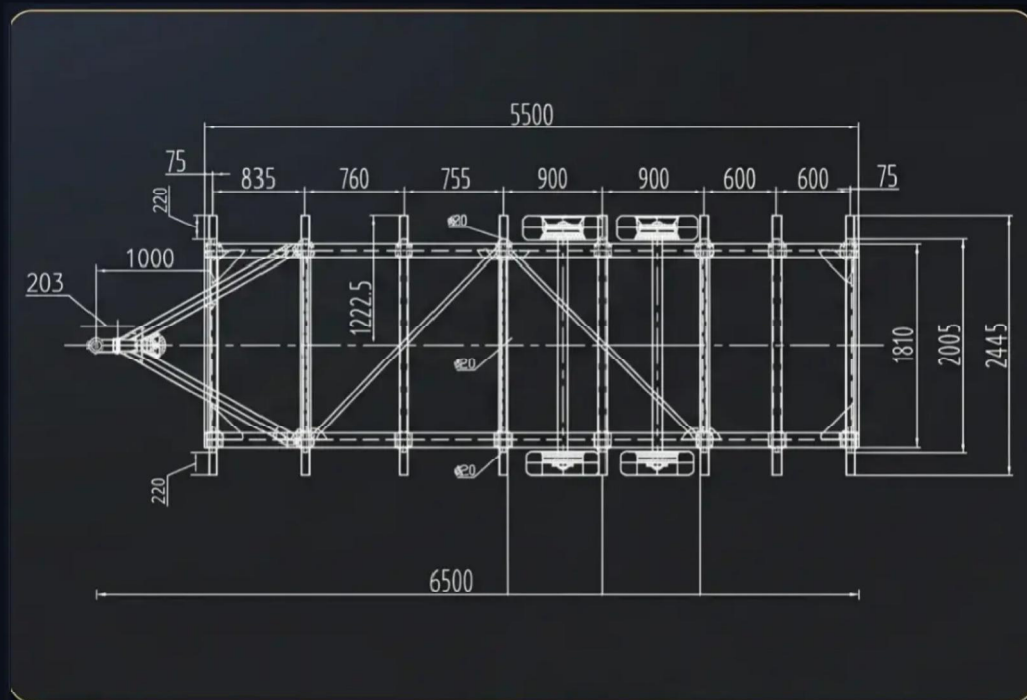
松華シャーシ 技術図面 — 特許取得済み
